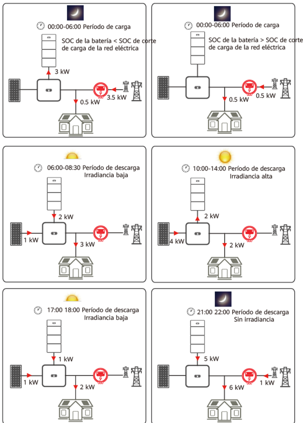
Figura 2-9 Ejemplo de TOU (carga de 00:00 a 06:00, y descarga de 6:00 a 24:00)
