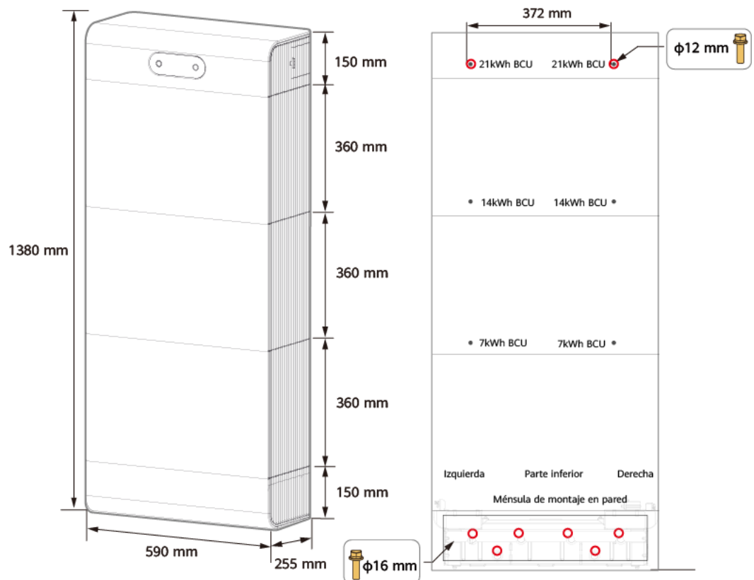
Figura 4-5 Dimensiones para el montaje en pared
