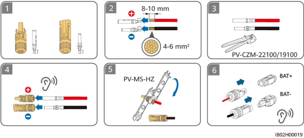
Figura 5-4 Conexión de los cables de entrada de CC
