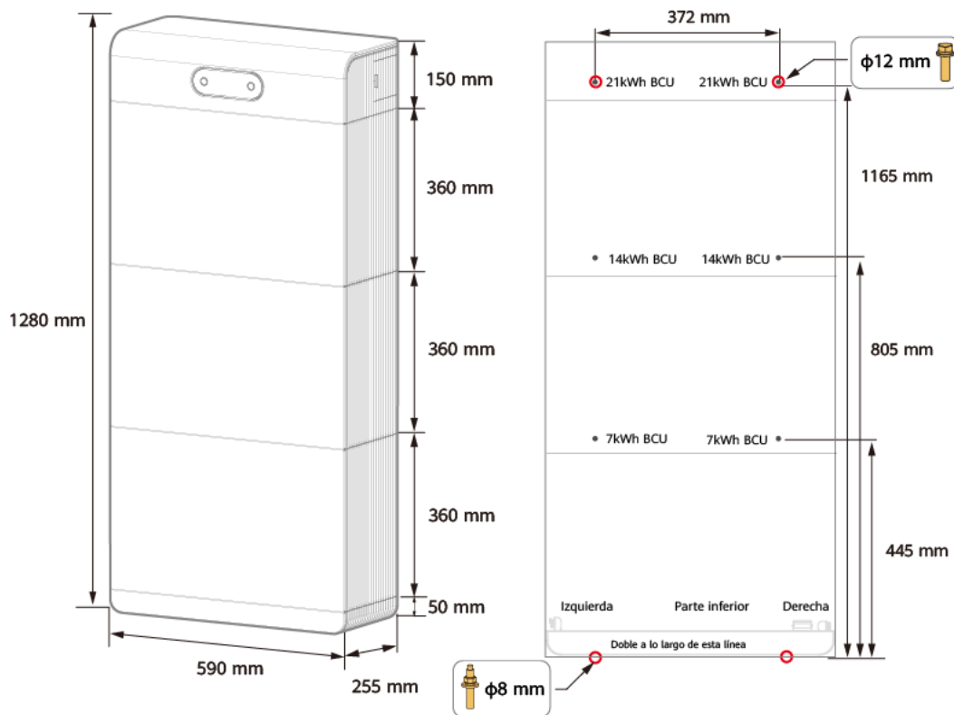
Figura 4-4 Dimensiones para el montaje en suelo
