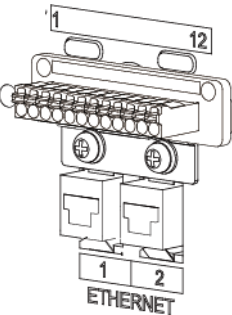
Figura 5-5 Puerto de señal
